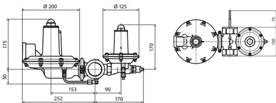
Rozměry [mm]
